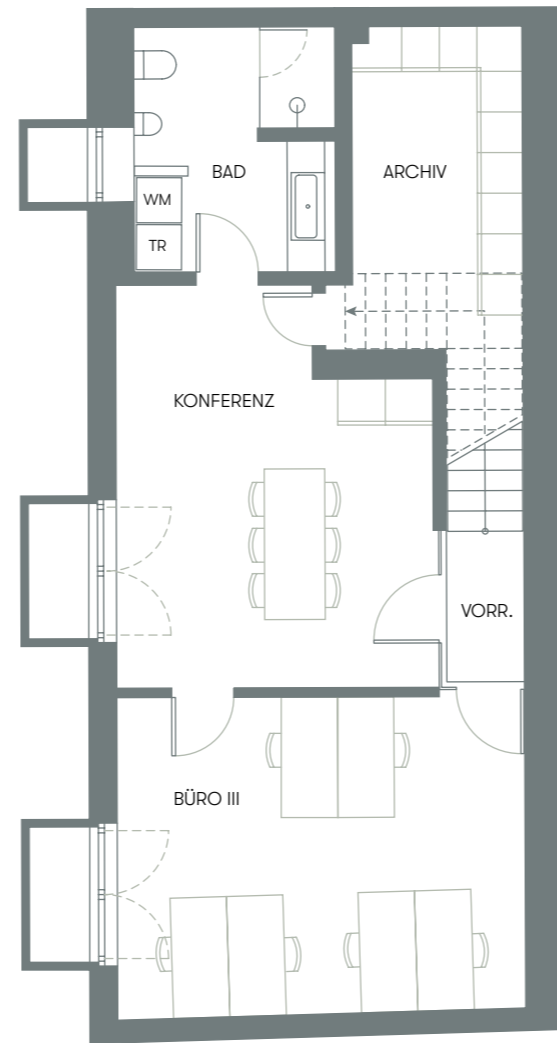
UNTERGESCHOSS
