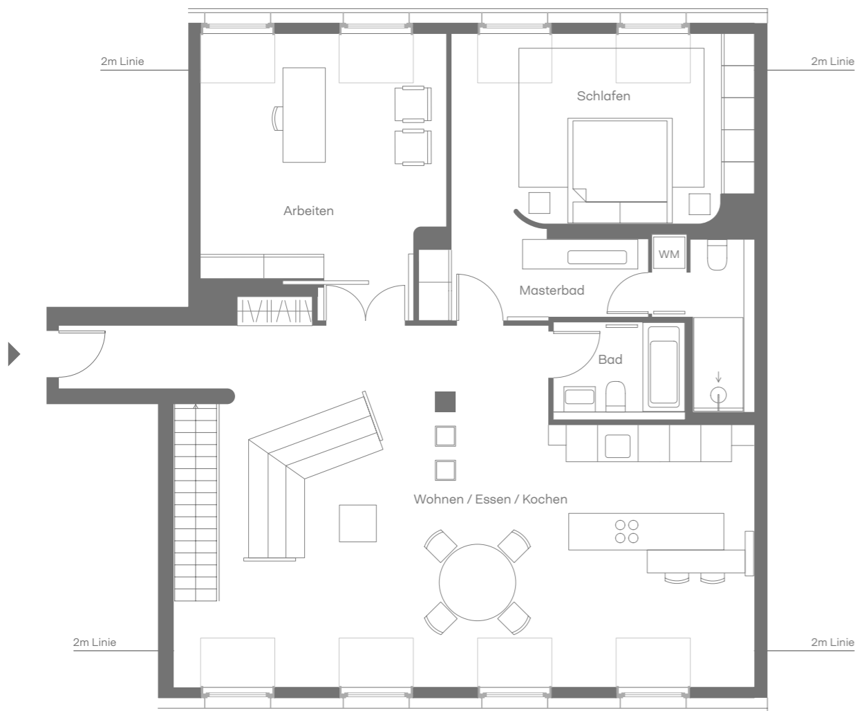
Dachgeschoss
